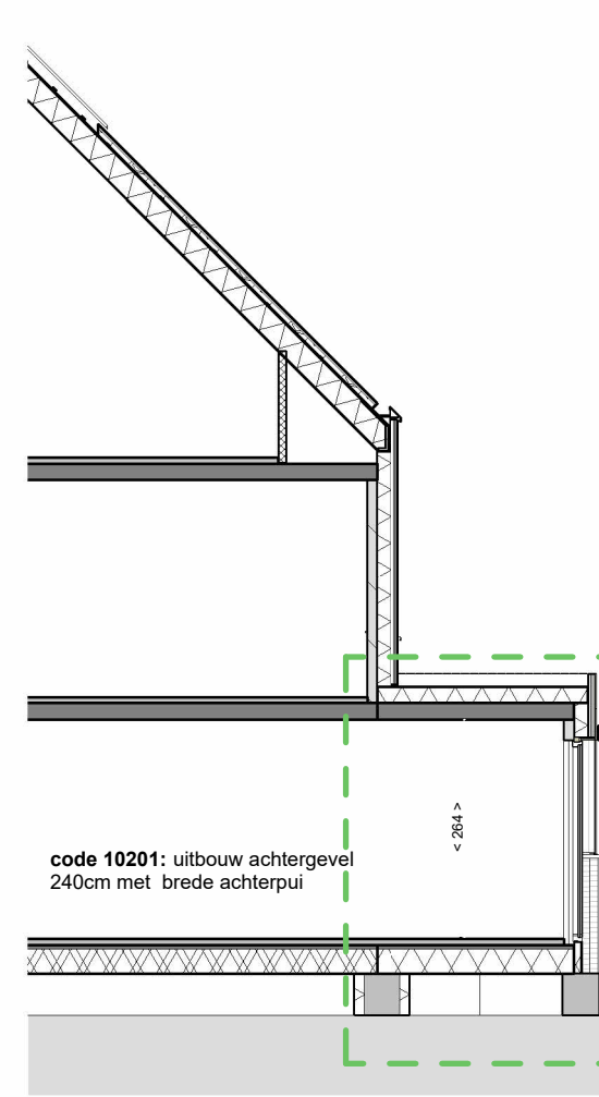
doorsnede
